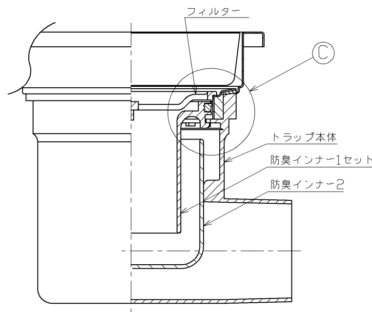
トラップ詳細図 (1:2)
