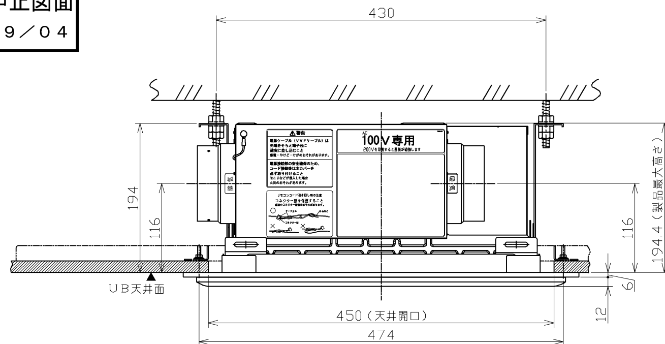
天井取付図
