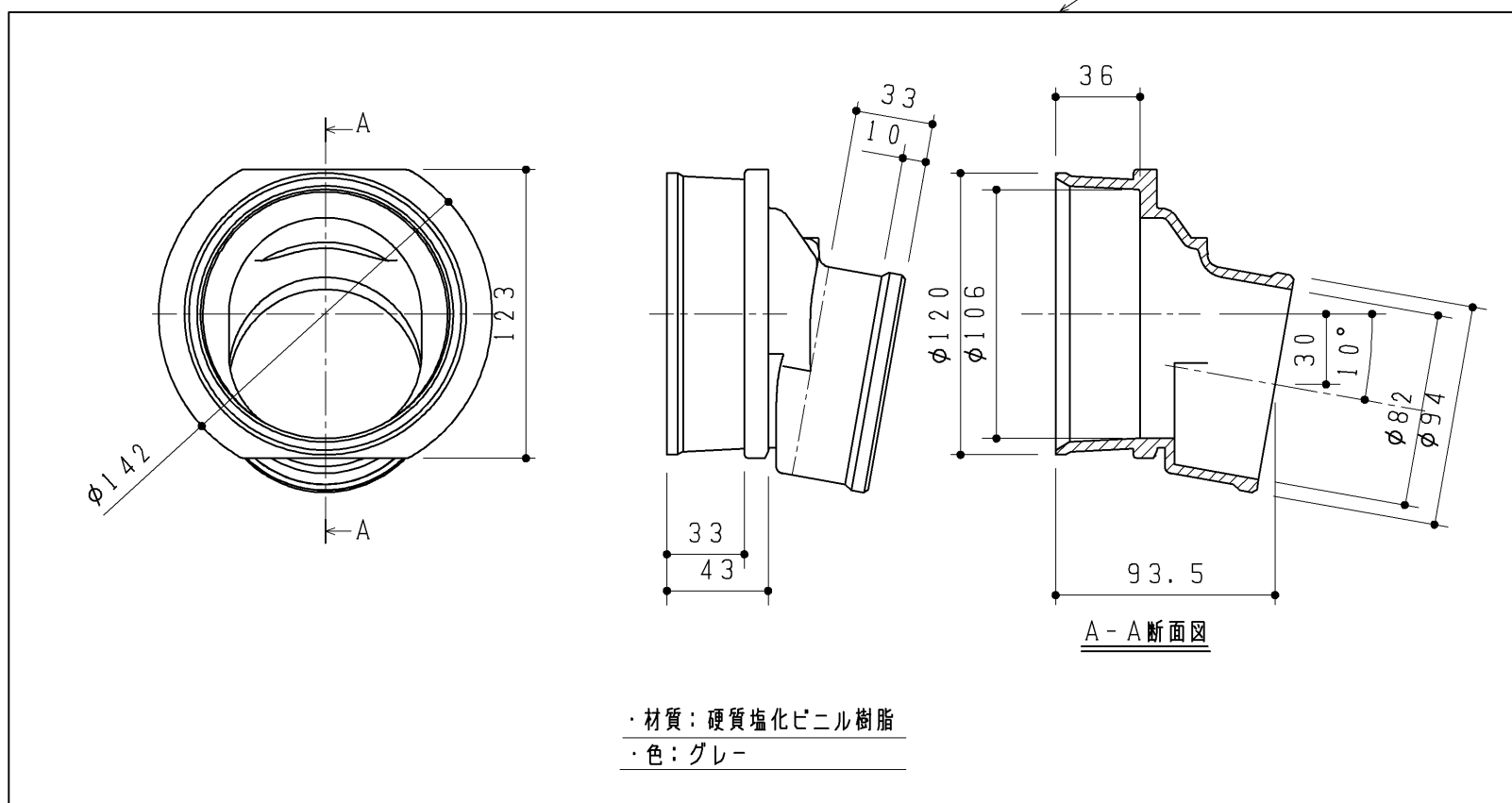
排水ジョイント
