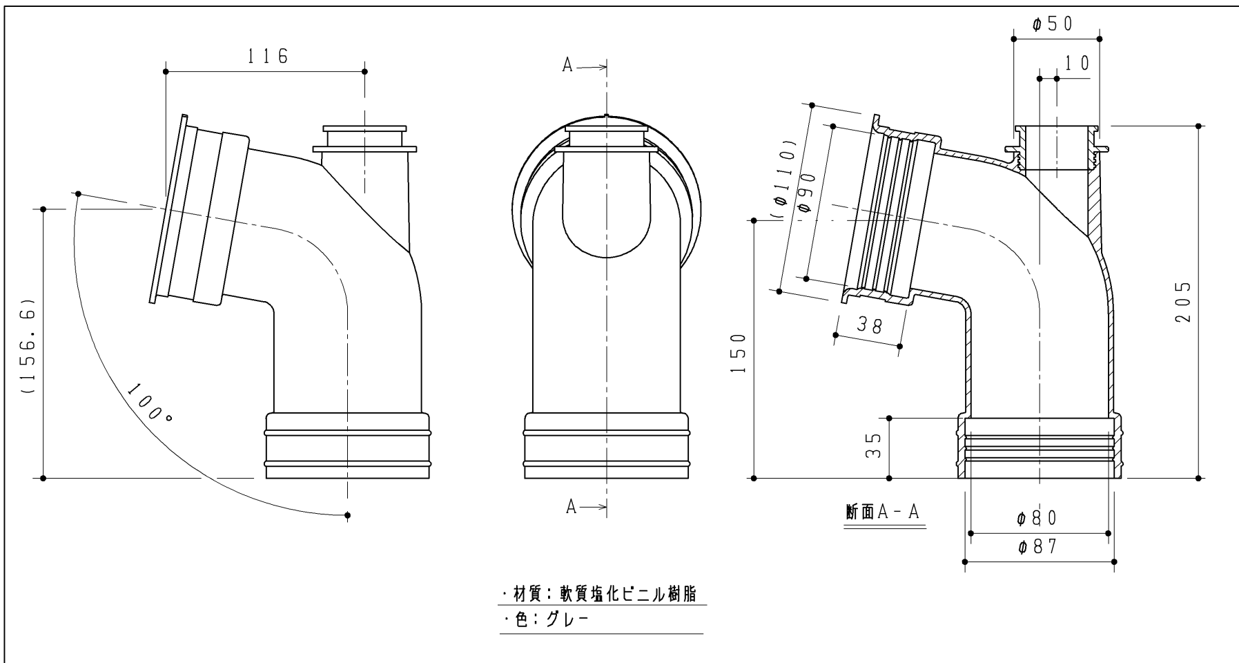
排水ソケット
