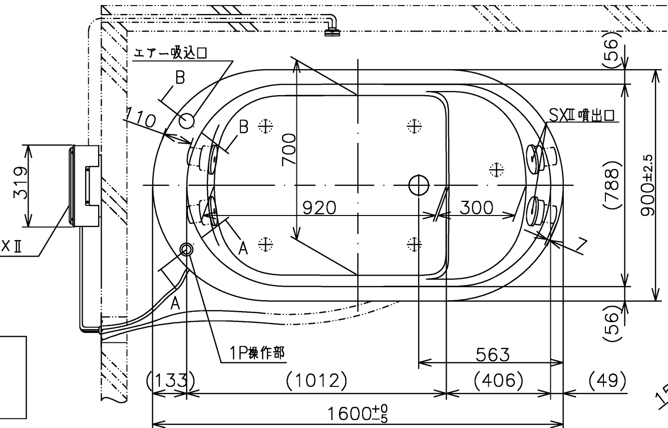
断面B-B(1:5)
