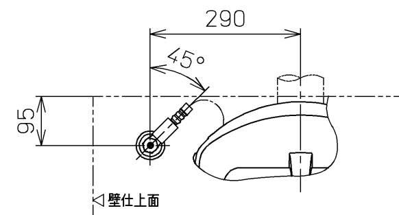
平面图
