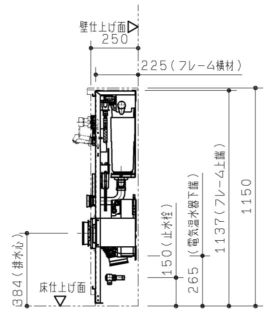
R 視図
