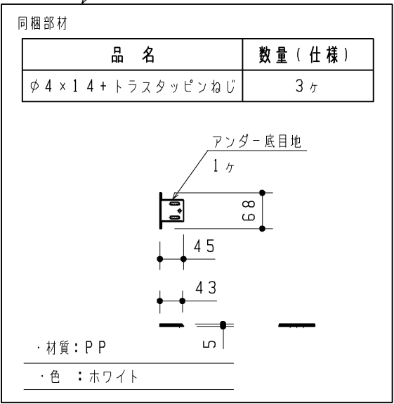
アンダー底目地セット 1セット
