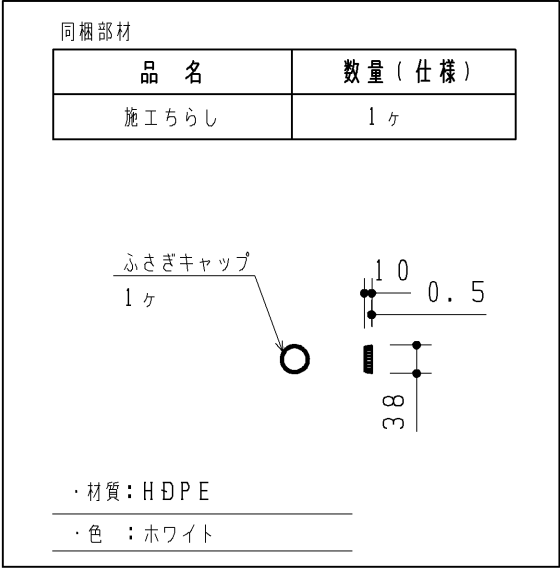
ふさぎキャップセット (φ35用) 1セット
