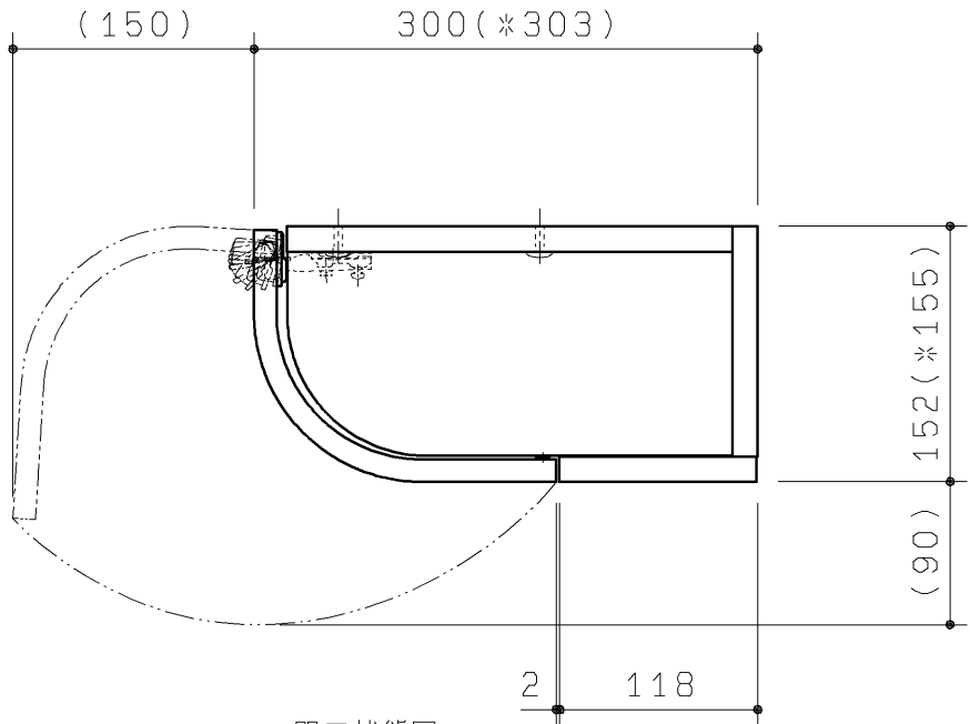
開口状態図
