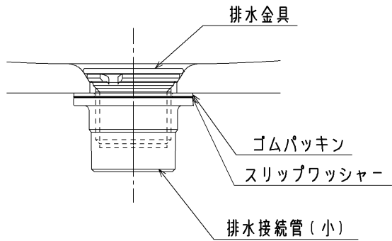
B 部詳細図 ( S = 1 : 1 )
