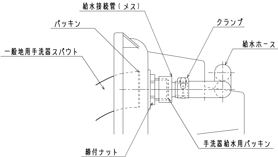
D 部詳細図 ( S = 1 : 1 )
