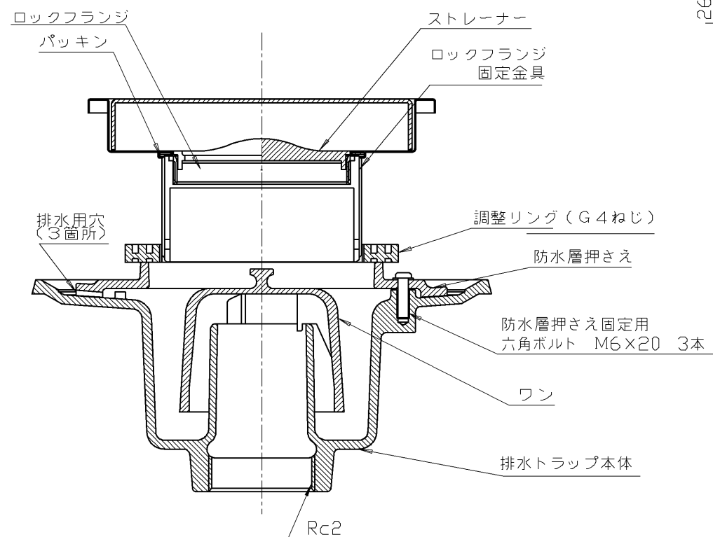
B-B断面 (尺度 フリー)
