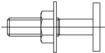
W5/16 山18×5.5 \phi 8.5 \times \phi 22 \times 1.2 各2ヶ
