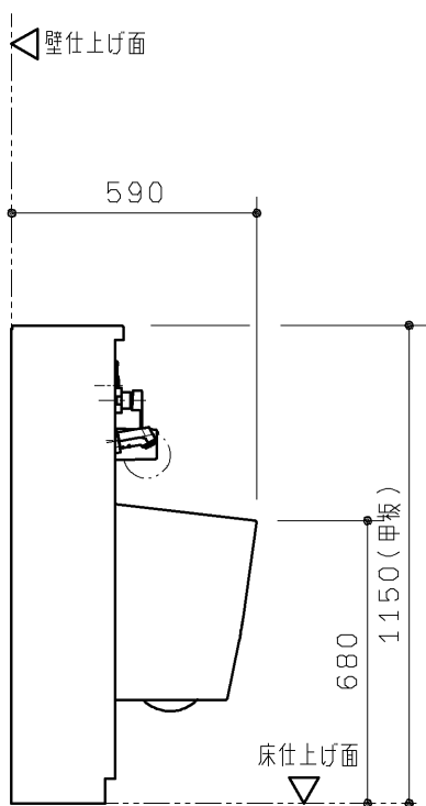
B矢視図
