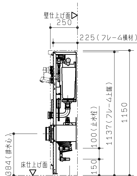
R 視図
