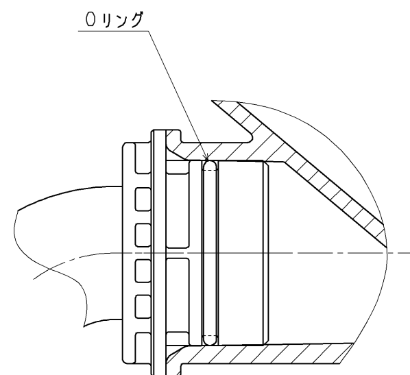
A - A (S = 1 : 1)
