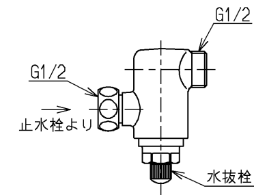
逆止弁ユニット(2ヶ入り)
