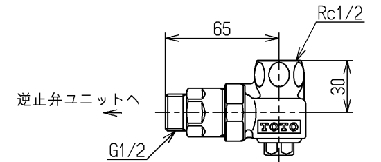
止水栓部(2ヶ入り)
