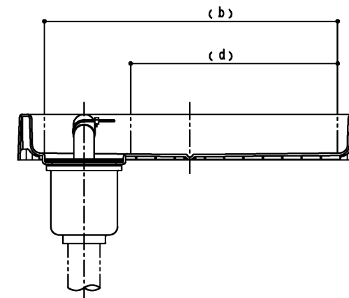
断面B-B
