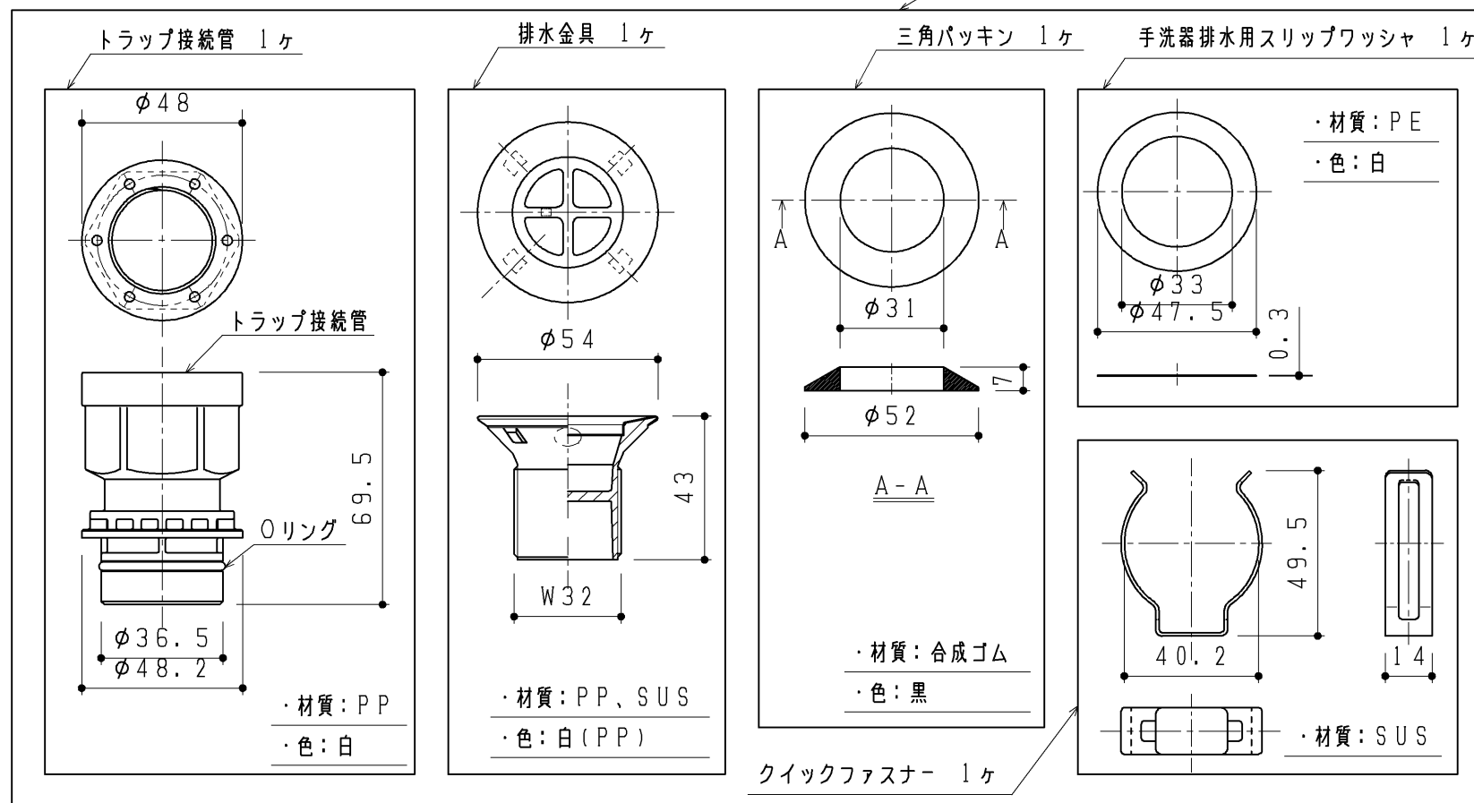
排水金具セット
