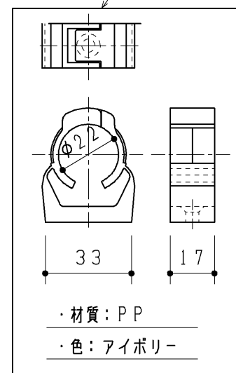
給水管支持材 2ヶ
