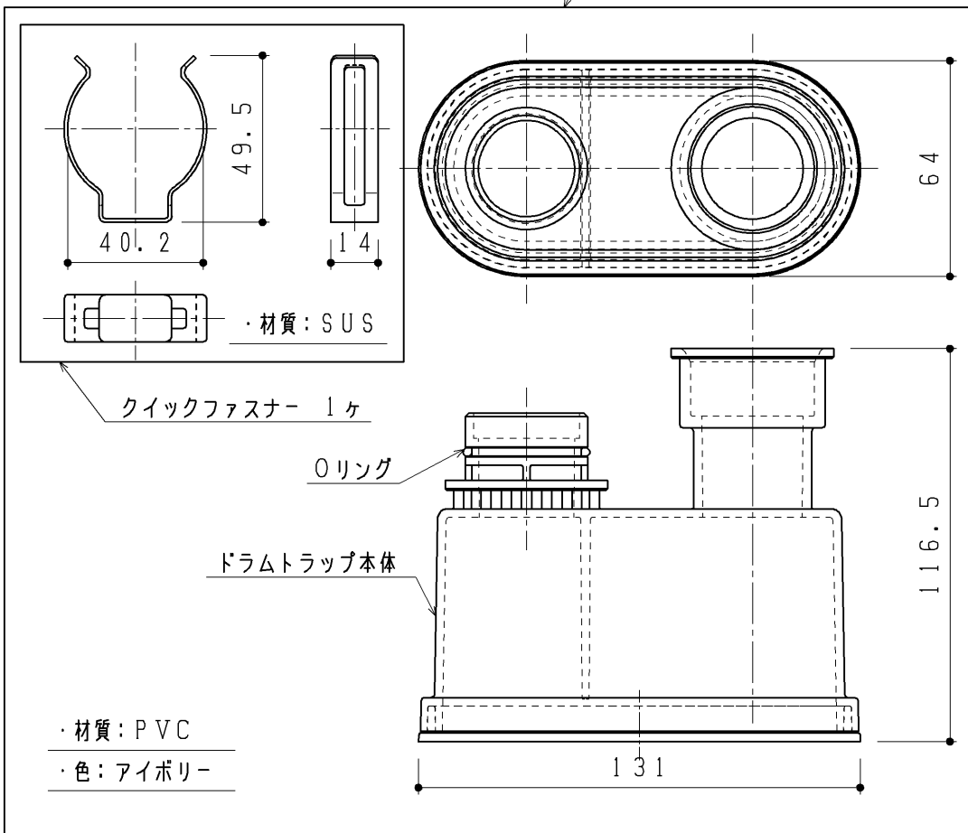
排水金具セット
