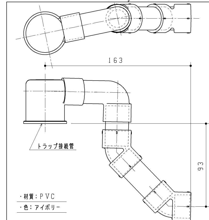
手洗排水ホースセット (床排水)
