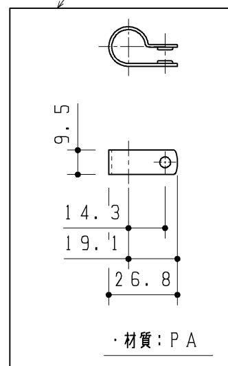
ホースクランプ 3ヶ
