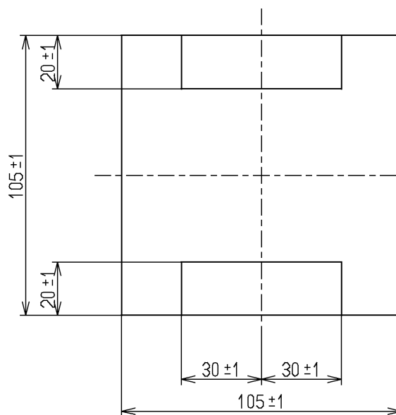
パネル壁の穴開け加工寸法
