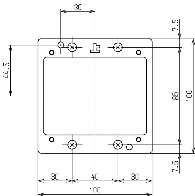
取付板部詳細図
