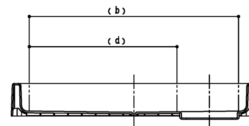
断面B-B
