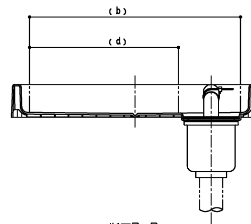
断面B-B
