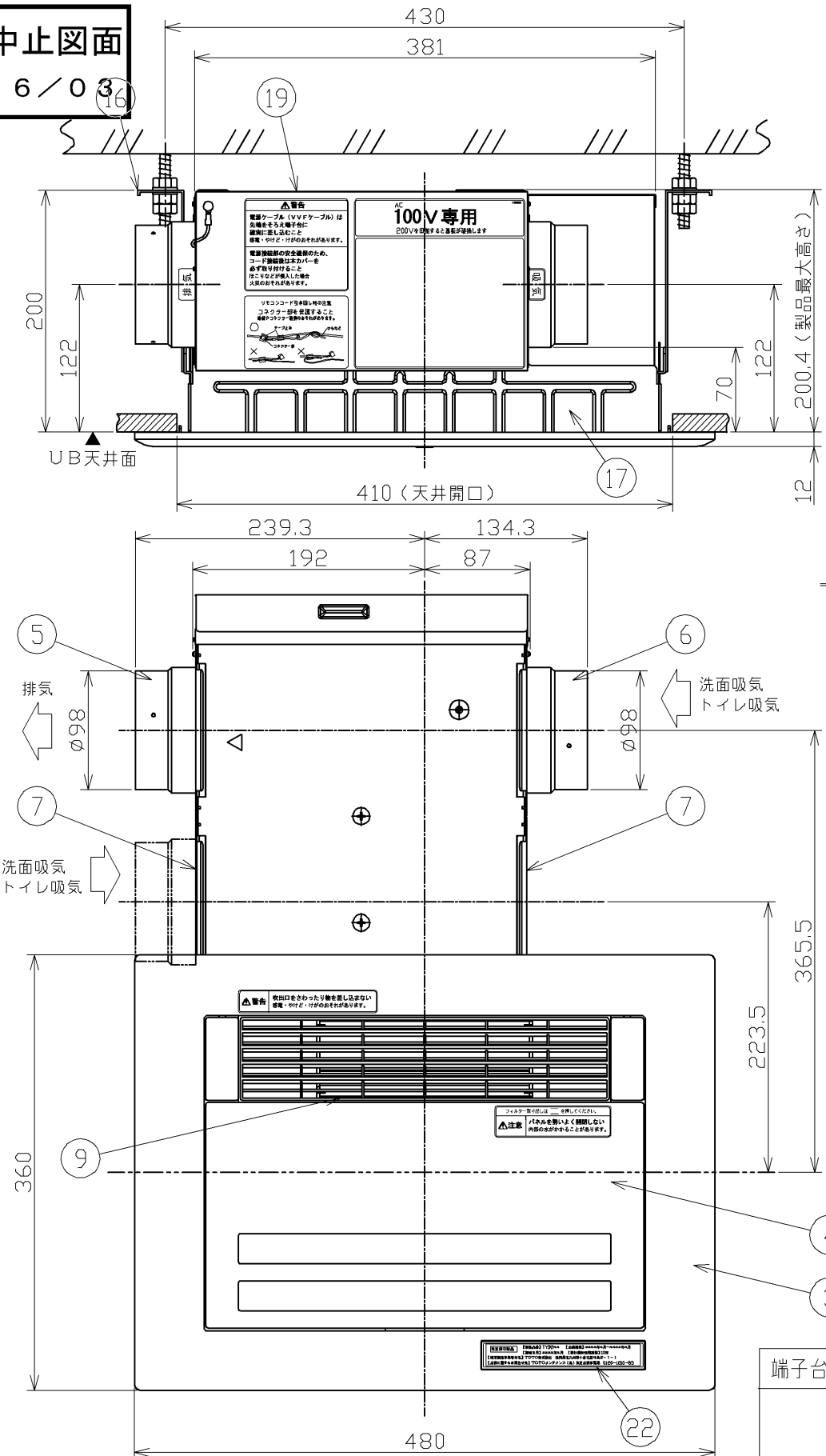
天井取付図 (1:5)
