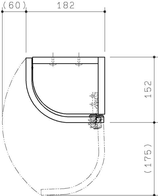
開口状態図
