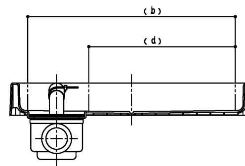
断面B-B
