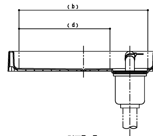
断面B-B
