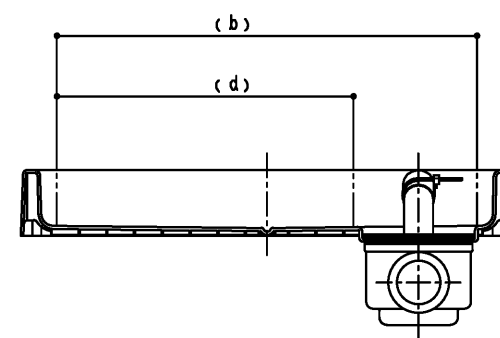
断面B-B
