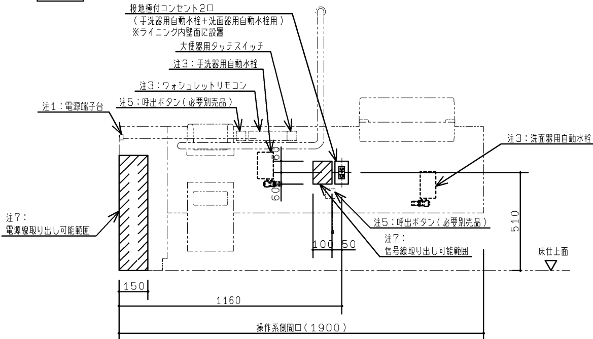
操作系部
