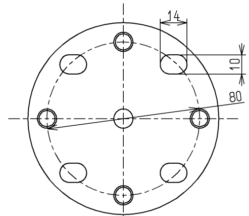
取付座詳細(1:2)
