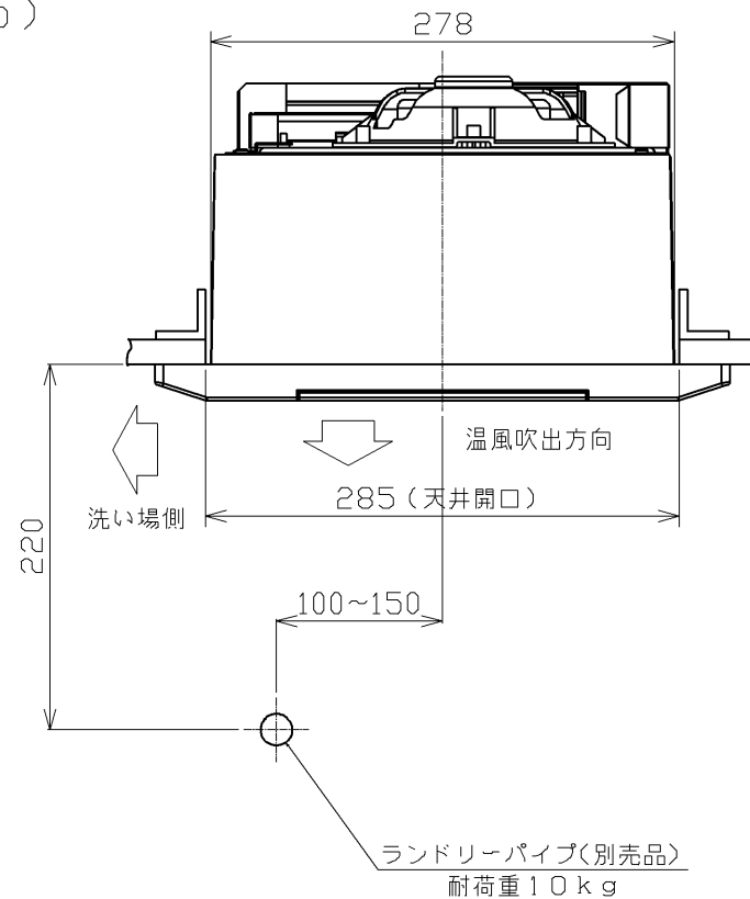
天井取付図 (1:5)
