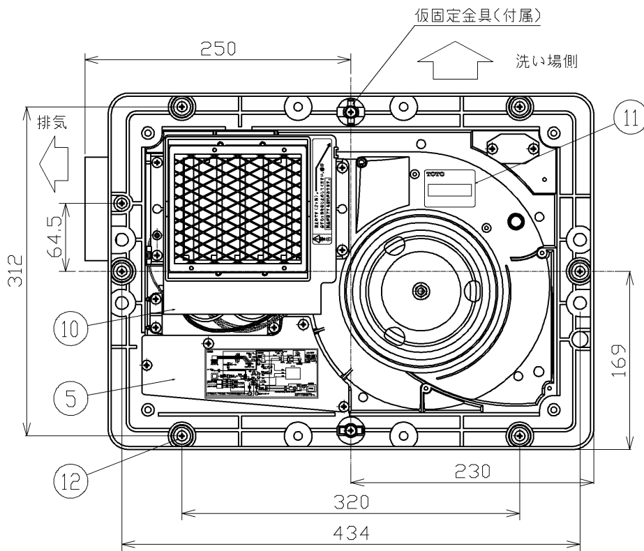
天井取付図 (1:5)
