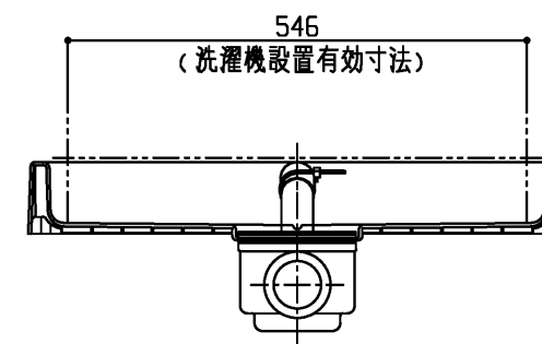
断面B-B
