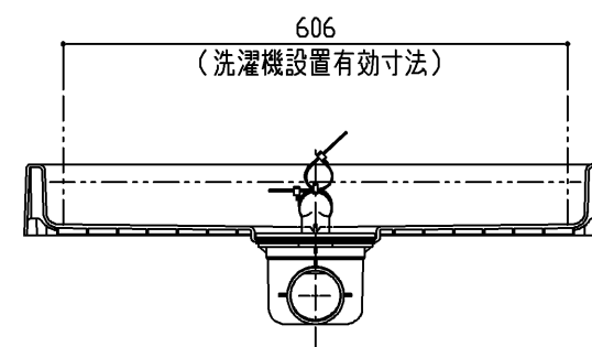
断面B-B
