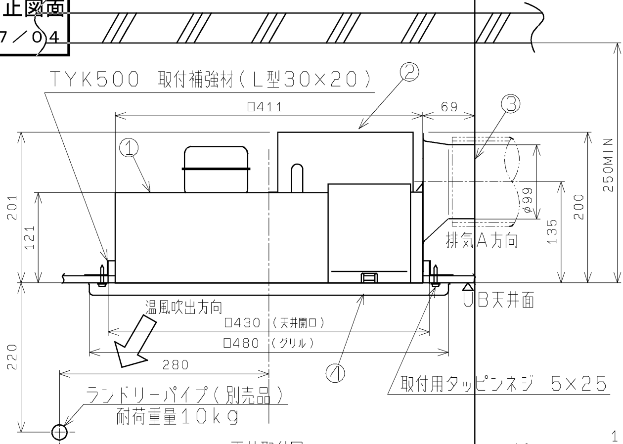
天井取付図
