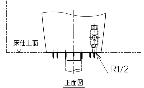
床給水仕様の場合
