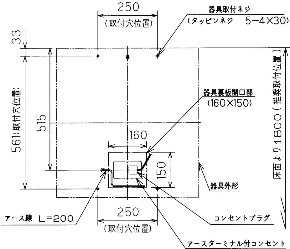
器具取付要領 (S=1/10)
