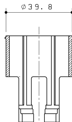
断面C-C
