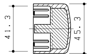
断面B-B
