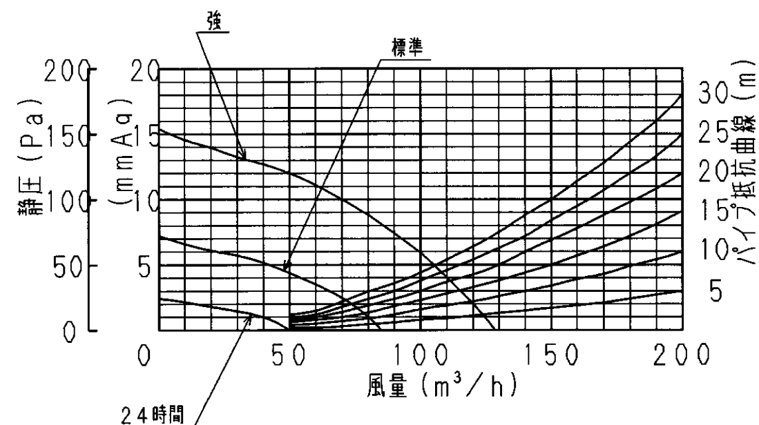
静圧風量特性曲線
