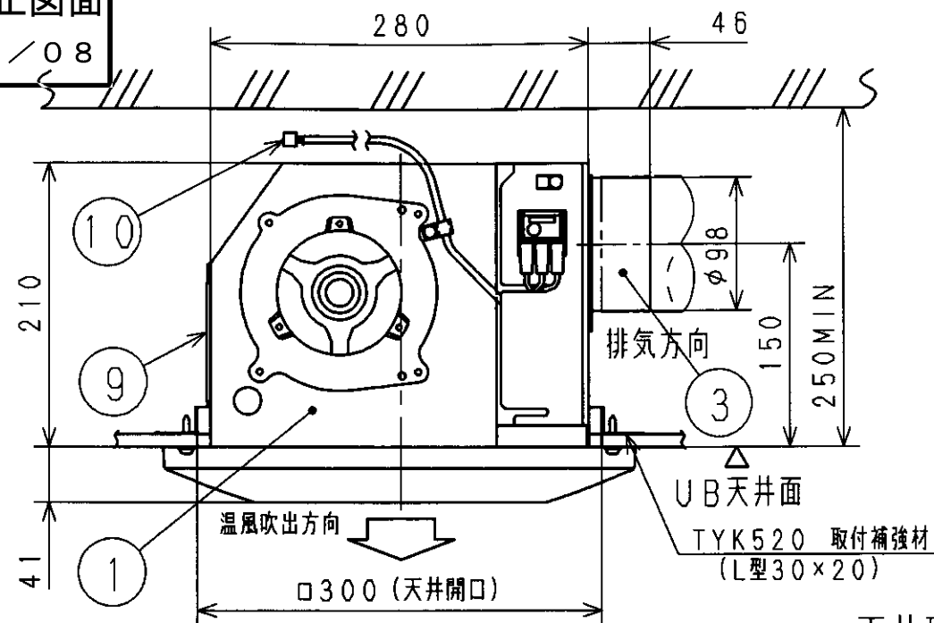
天井取付図 (1:5)
