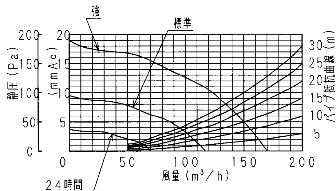
静圧風量特性曲線
