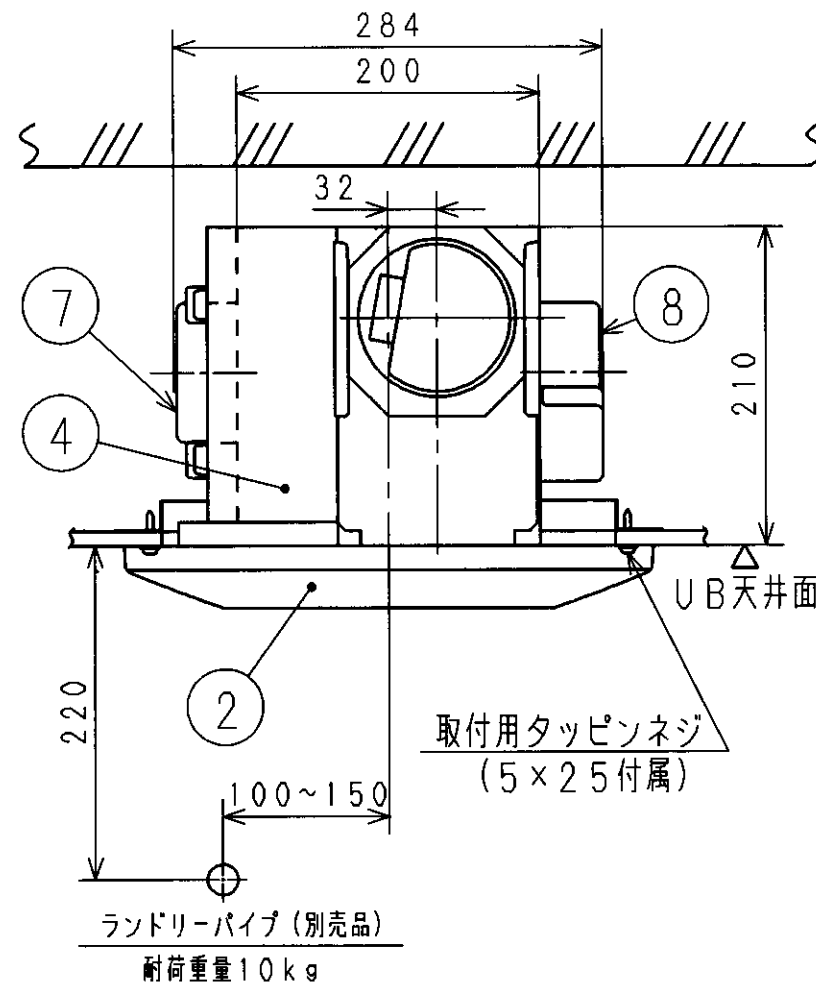
天井取付図 (1:5)
