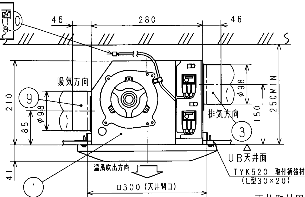
天井取付図 (1:5)
