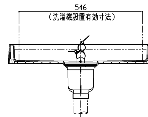
断面B-B
