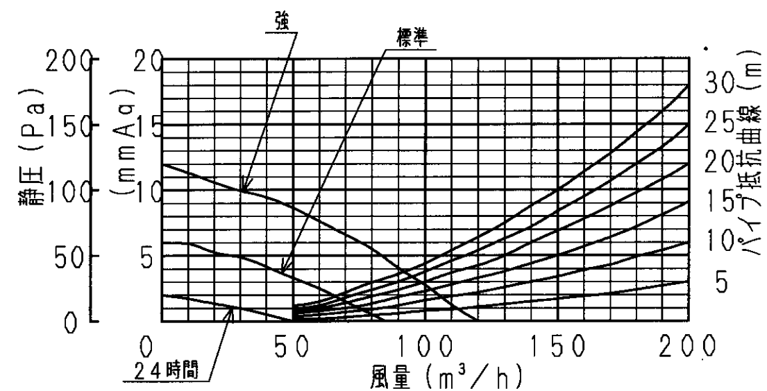
靜壓風量特性曲線
