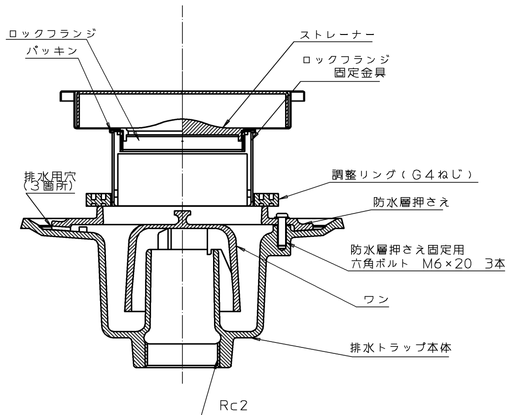
B-B断面（尺度 フリー）
