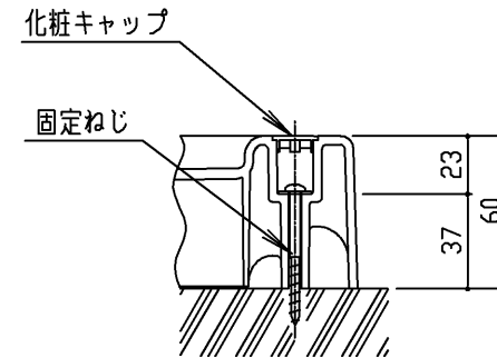
固定部詳細(尺度フリー)
