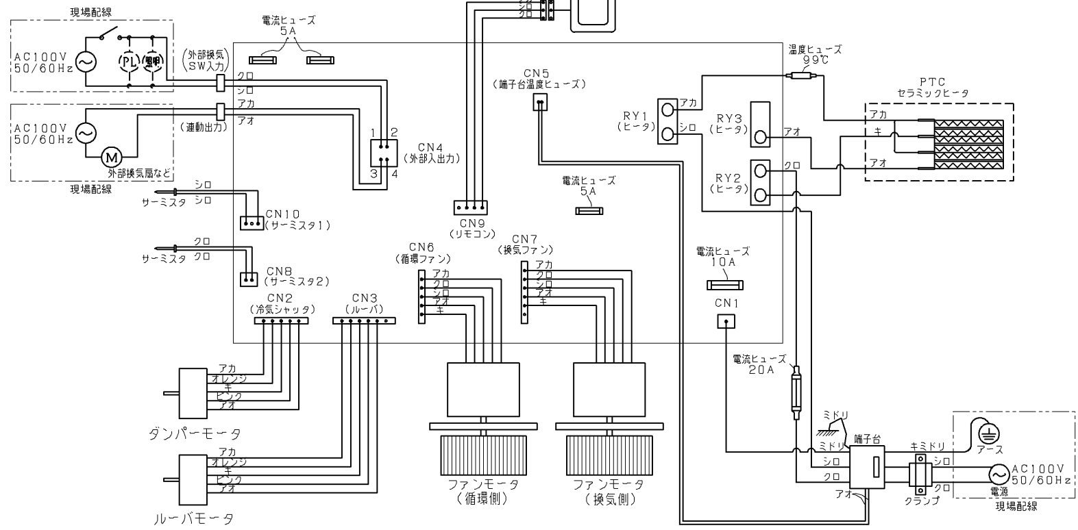
＜結線図＞
