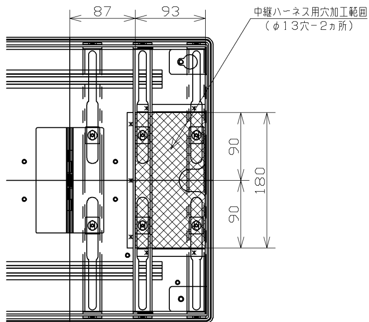
中継ハーネス用穴加工範囲
