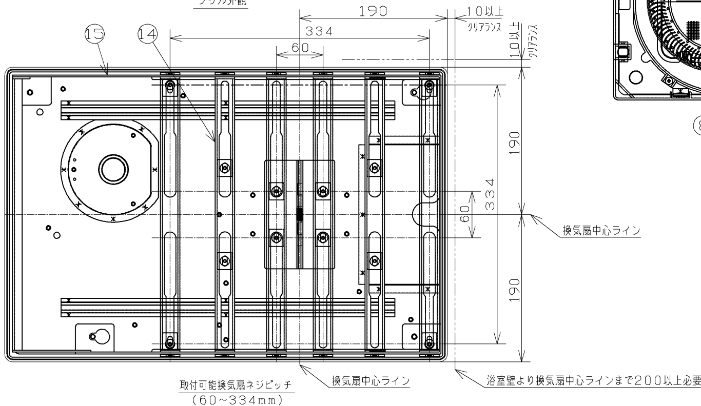
グリル外観
