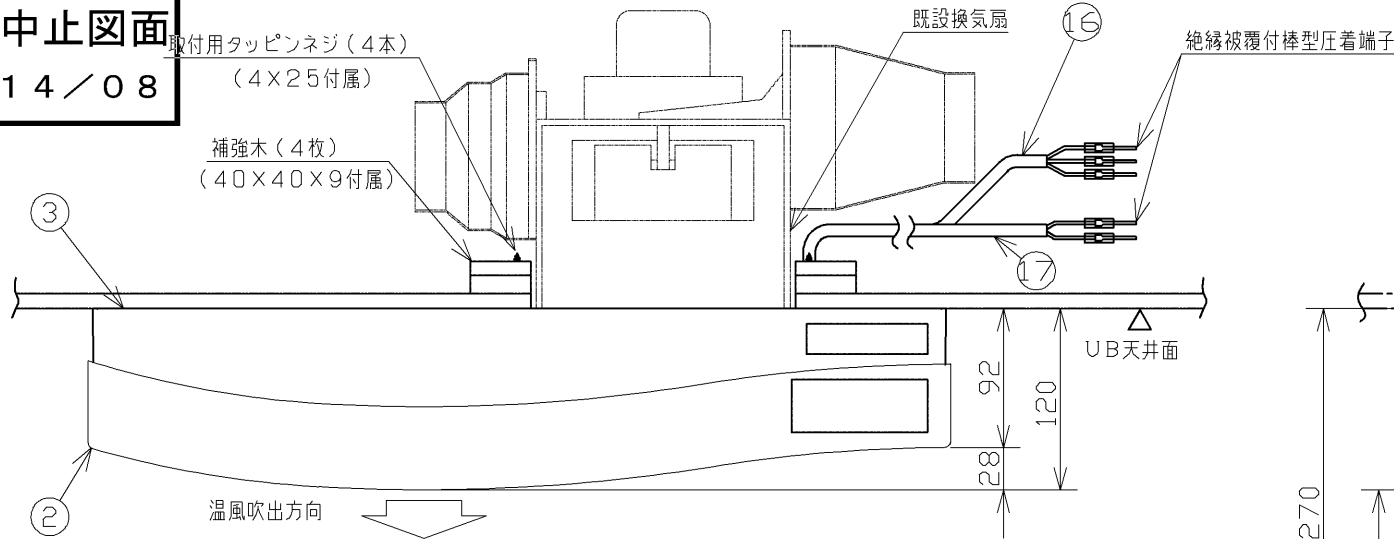
天井取付図
