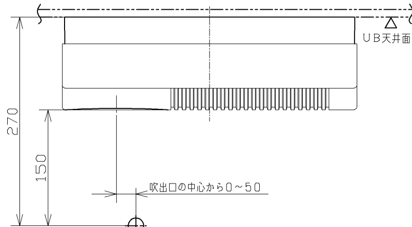
ランドリーパイプ取付推奨位置 (別売品) 耐荷重量10kg
