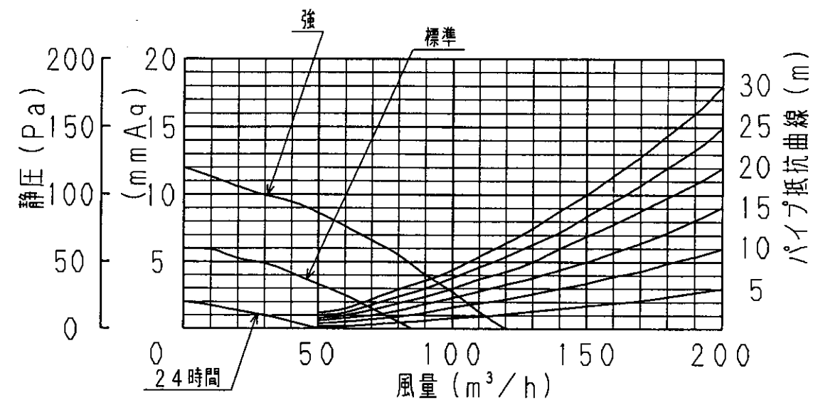
静圧風量特性曲線
