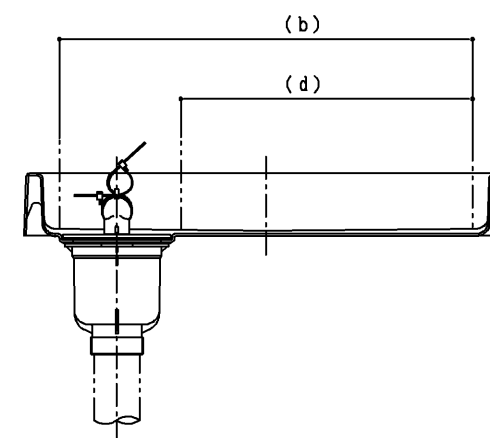
断面B-B
