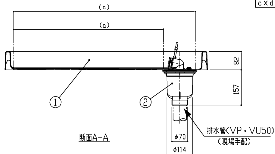
洗濯機設置有効寸法組合せ
