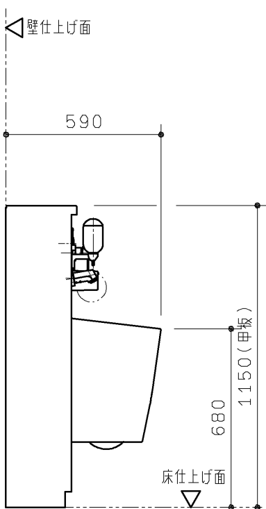
B矢視図
