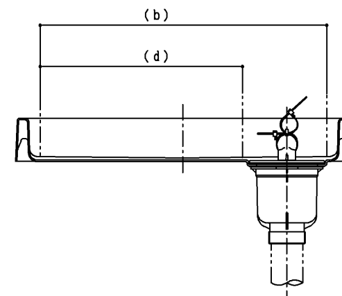
断面B-B
