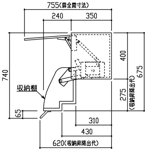
昇降ウォール詳細寸法（側面図）
