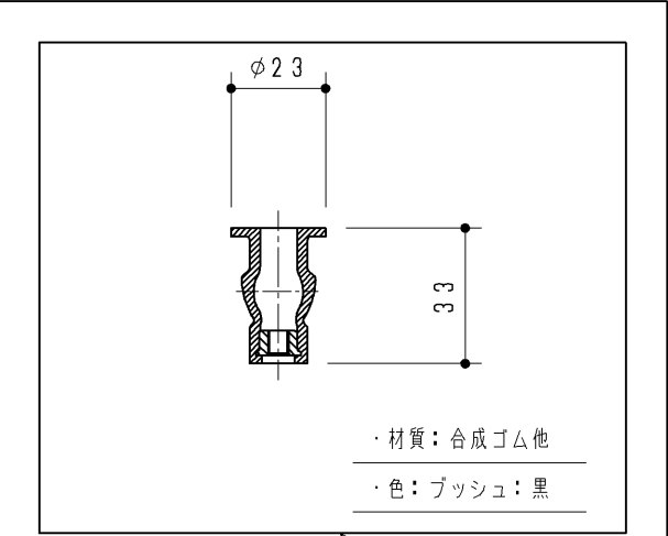
固定ブッシュ 2ヶ
