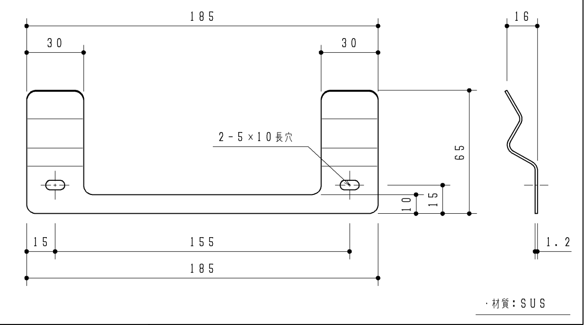
手洗器固定金具 1ヶ
