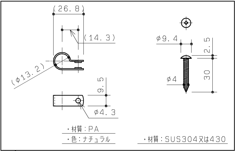
ホースクランプ 1ヶ φ4×30+トラスタッピンねじ 1ヶ
