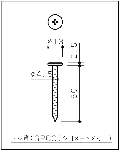
特殊+4.5×50TPねじ（焼き入れ品） 2ヶ
