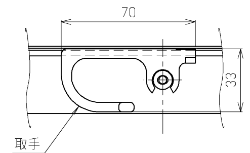
B-B断面詳細図 (1:2)
